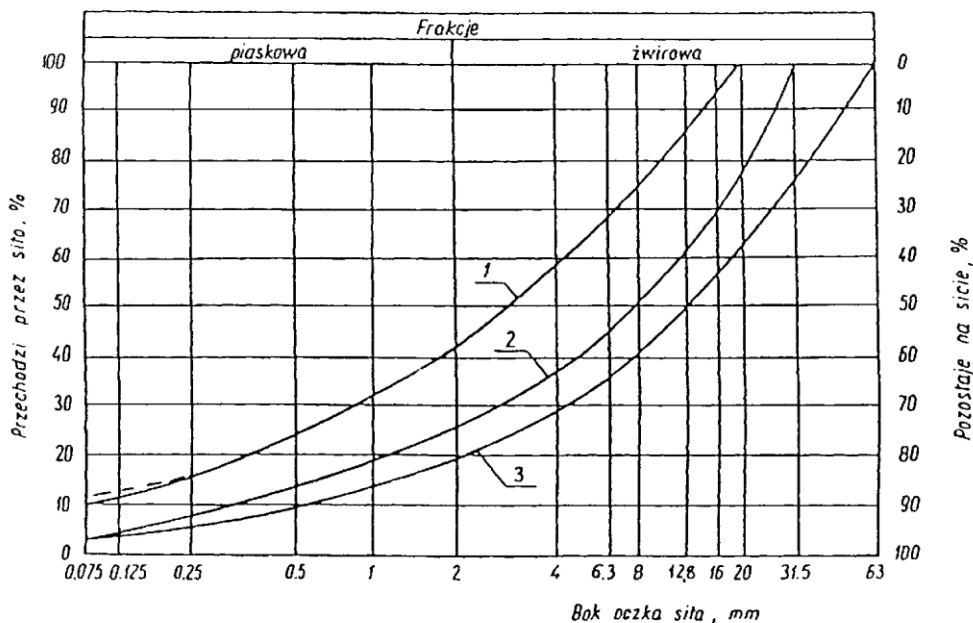
Rysunek 1. Pole dobrego uziarnienia a kruszywo przewidziane na podbudowę wykonywane metodą stabilizacji mechanicznej
