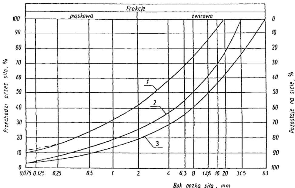
Rysunek 1. Pole dobrego uziarnienia a kruszyw przeznaczonych na podbudowy wykonywane metodą stabilizacji mechanicznej
