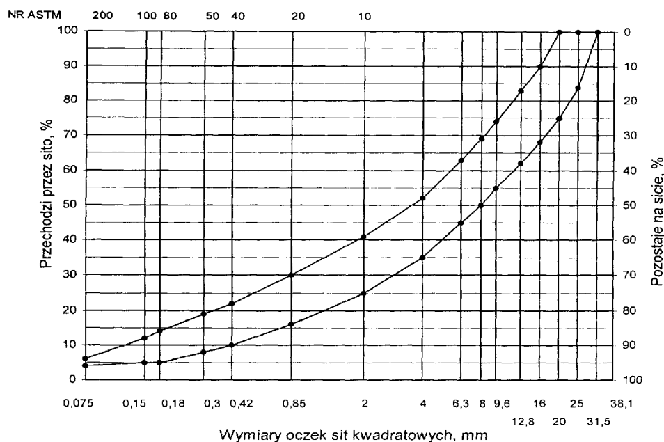
Rys. 1. Krzywe graniczne uziarnienia mieszanki mineralnej BA od 0 do 20 mm do warstwy wiążącej o obciążeniu ruchem KR4
