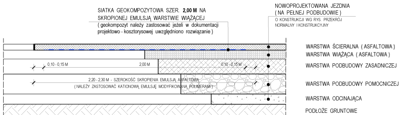
Rys. 2. Konstrukcja połączenia nowego poszerzenia i starej nawierzchni
