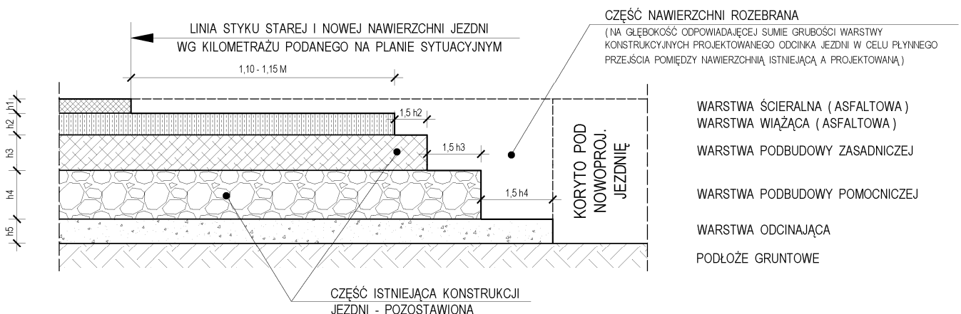
Rys. 2. Konstrukcja połączenia nowego poszerzenia i starej nawierzchni
