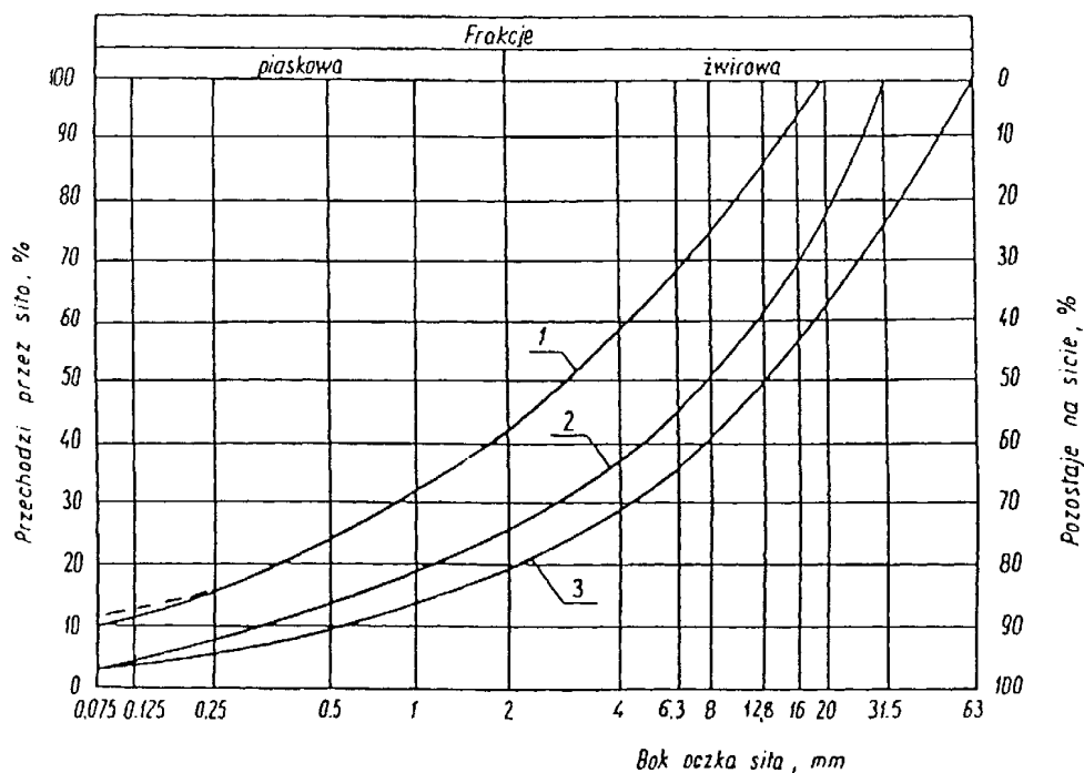
Rysunek 1. Pole dobrego uziarnienia kruszyw przeznaczonych na podbudowy wykonywane metodą stabilizacji mechanicznej 1-2 kruszywo na podbudowę zasadniczą (górną warstwę) lub podbudowę jednowarstwową 1-3 kruszywo na podbudowę pomocniczą (dolną warstwę)
